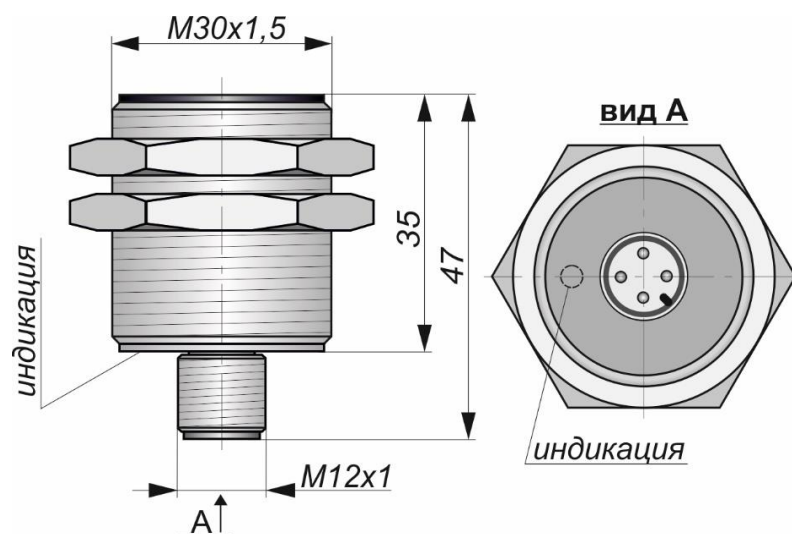
Габаритный чертеж
